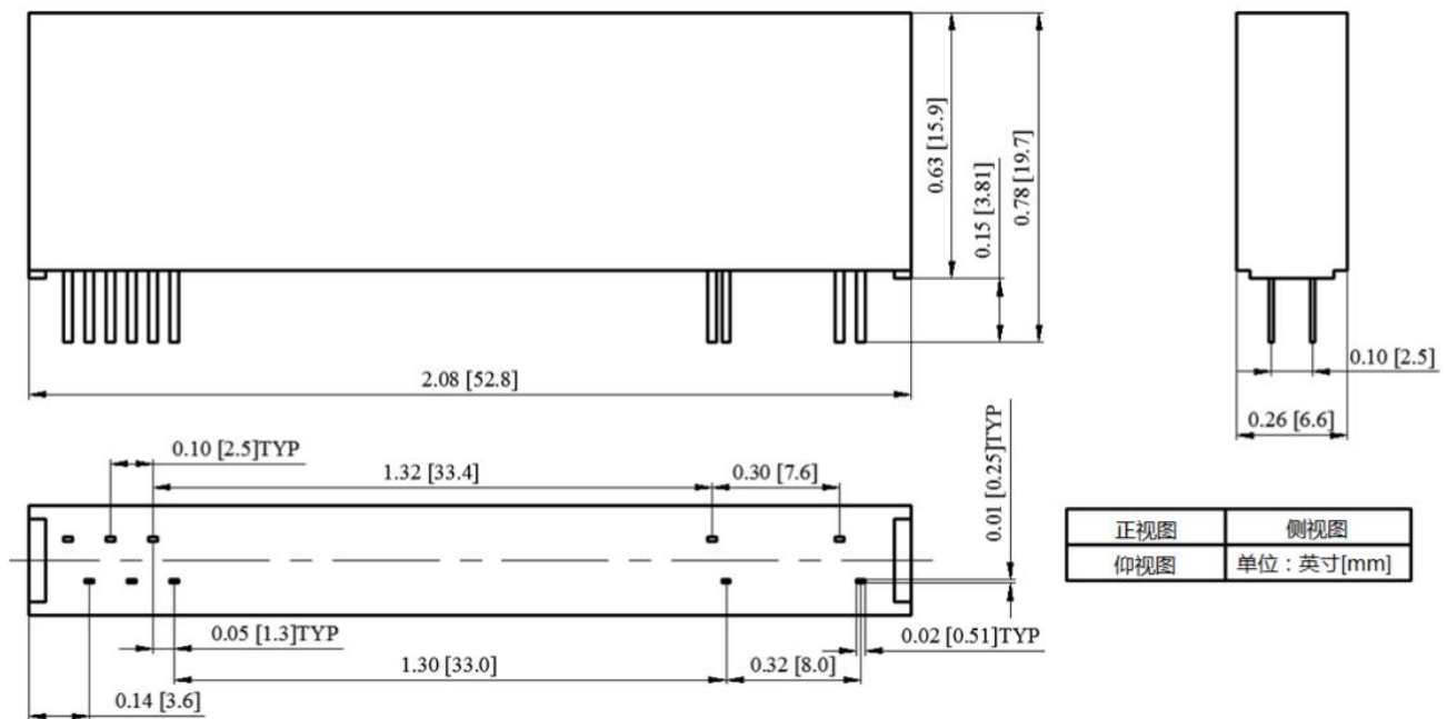
图 10. 2. AD202JNAIT 与 AD202KYAIT SIP 封装的尺寸
