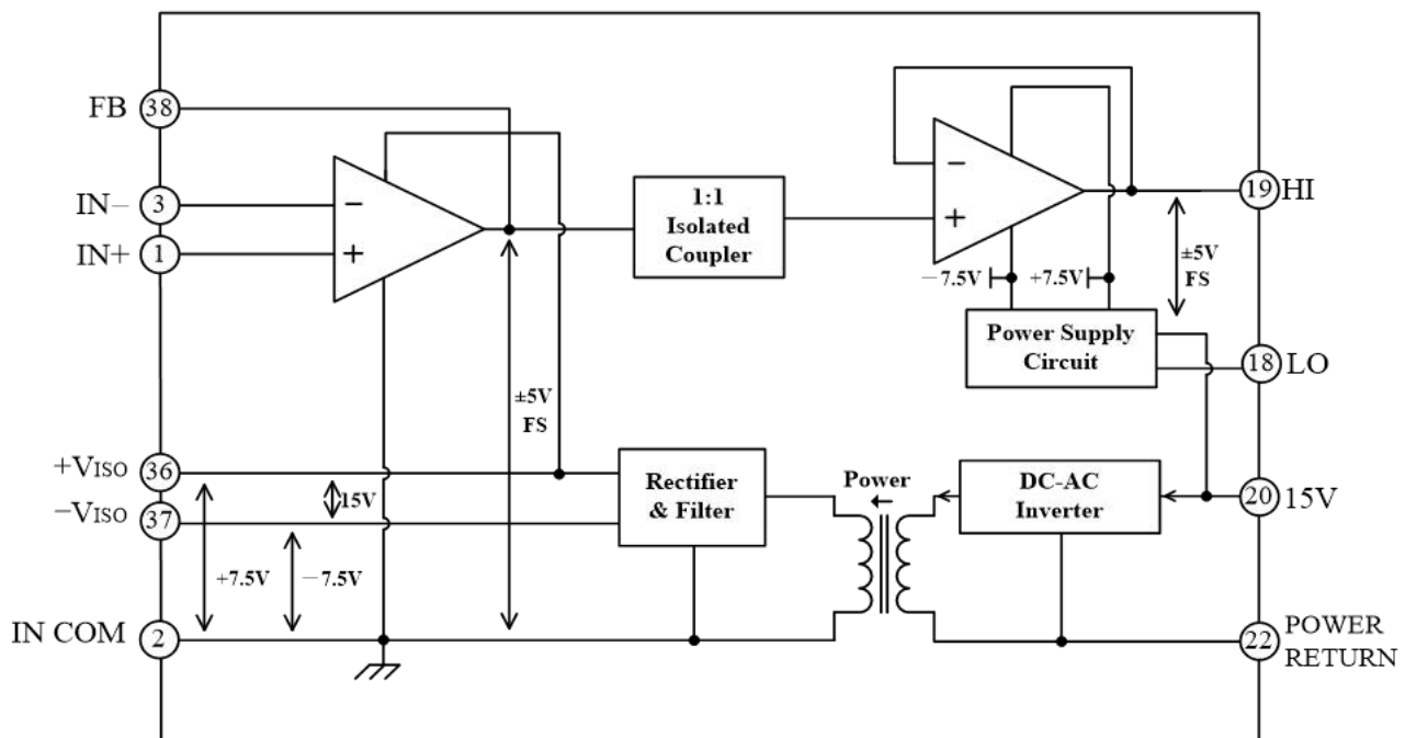
图 2. AD202KNAIT 的功能方框图
